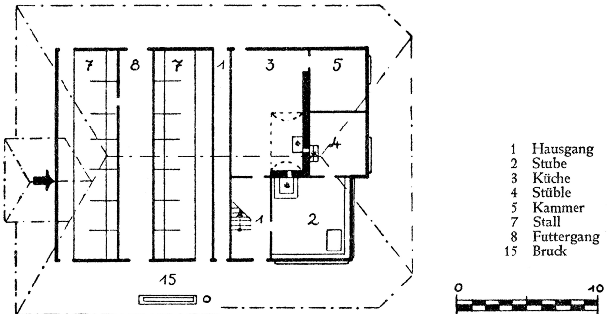
Figur 29. Grundrisse der jüngeren Form des Heidenhauses k Oberried-Dietenbach. Fushof. Erbaut 1754. Erdgeschoß.
